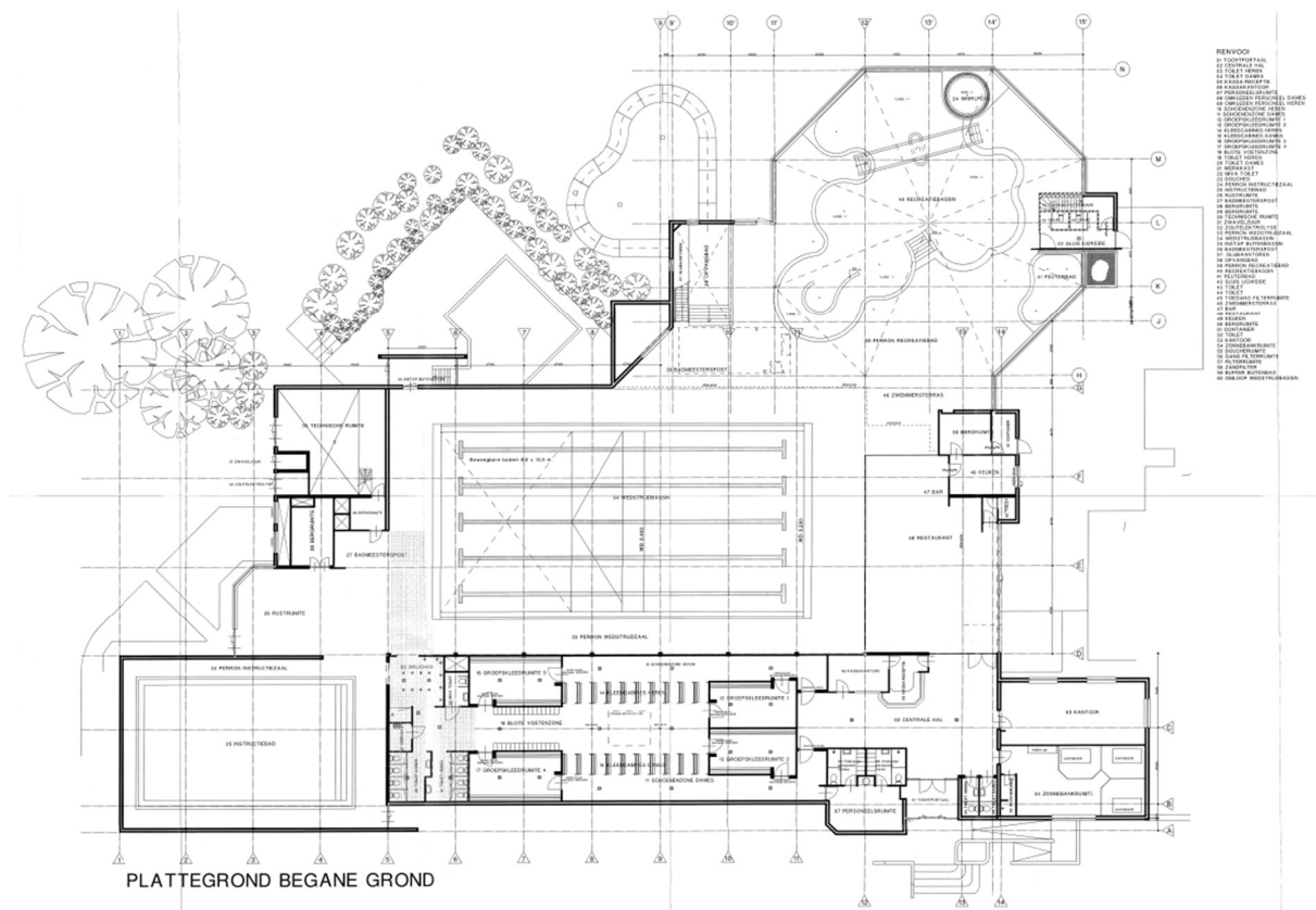
Figuur 1.1 Plattegrond BG zwembad Poelmeer - huidige situatie
